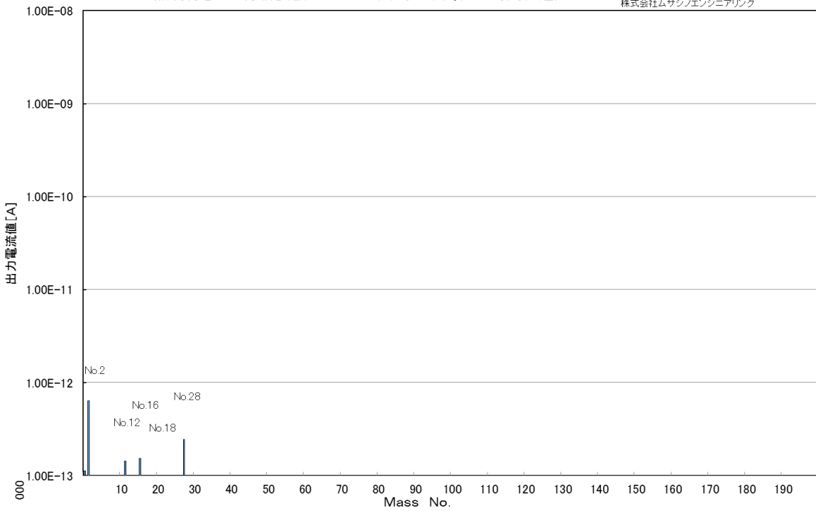
MVE-05H照明付きガス分析試験 マスピーークグラフ(本体 48時間経過)
