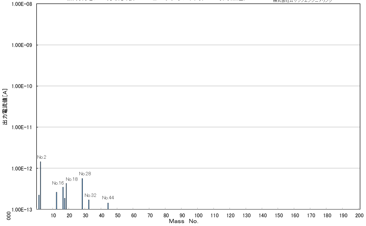
MVE-05H照明付きガス分析試験 マスピーークグラフ(本体 24時間経過)
