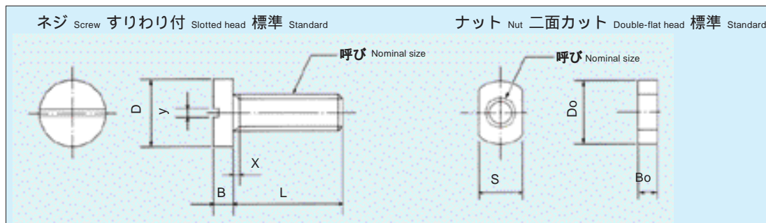
セラミックネジ Ceramic Screws
