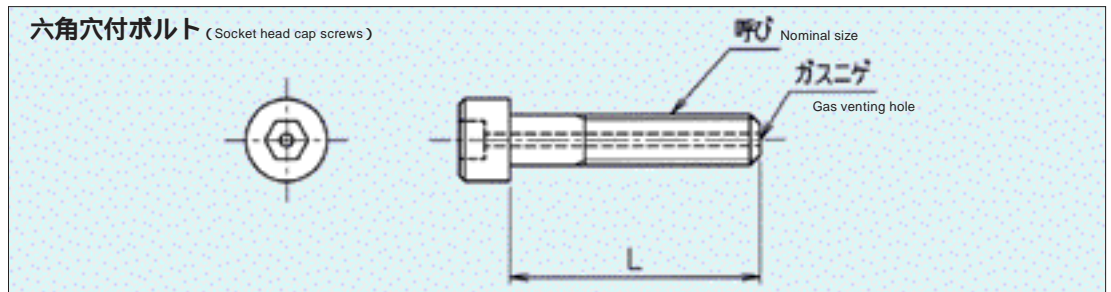
六角穴付きボルト主要・寸法及び価格 Socket head cap screws main dimensions and price
